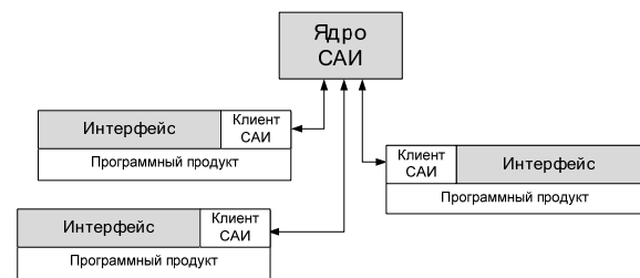
Рисунок 5 – Клиент серверная архитектура, включающая САИ
