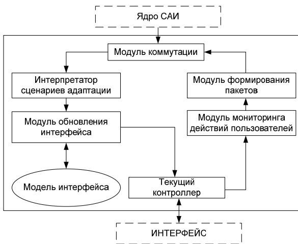
Рисунок 6 – Структура клиентской части САИ
