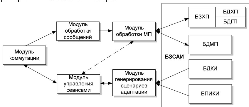
Рисунок 7 – Структура ядра САИ
