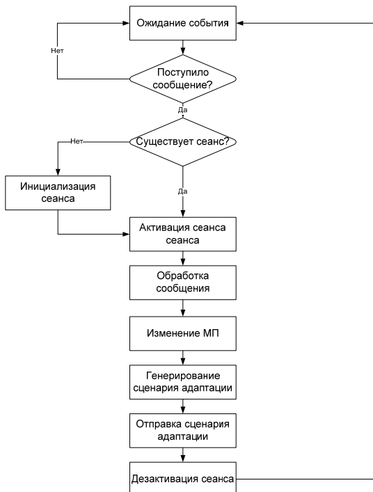
Рисунок 8 – Обобщенный алгоритм функционирования ядра САИ
