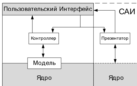
Рисунок 4 – Структура программного продукта с САИ
